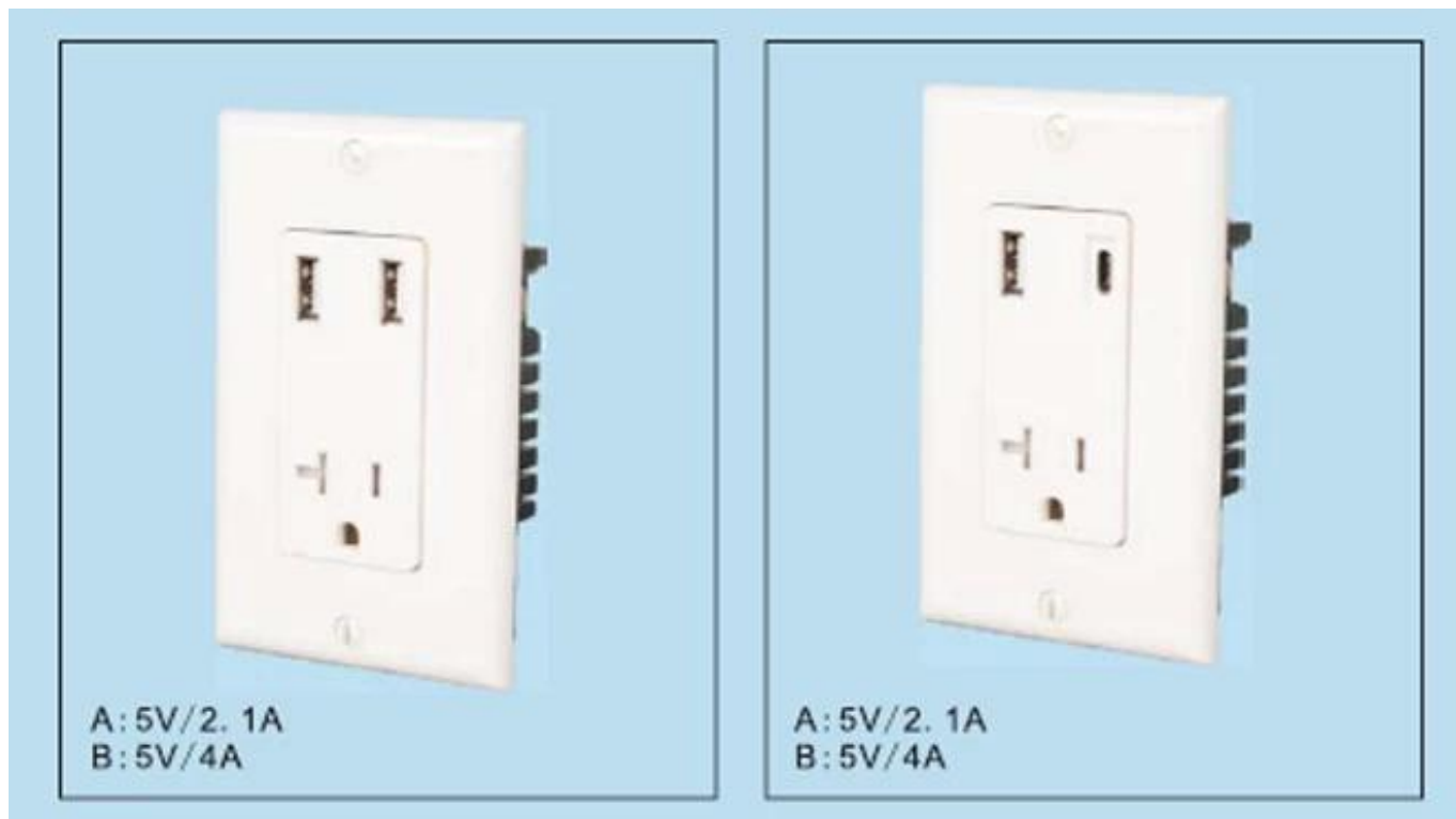
USB 插座 產品 照片
