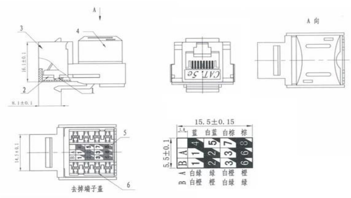
Cat5e Drawing:
